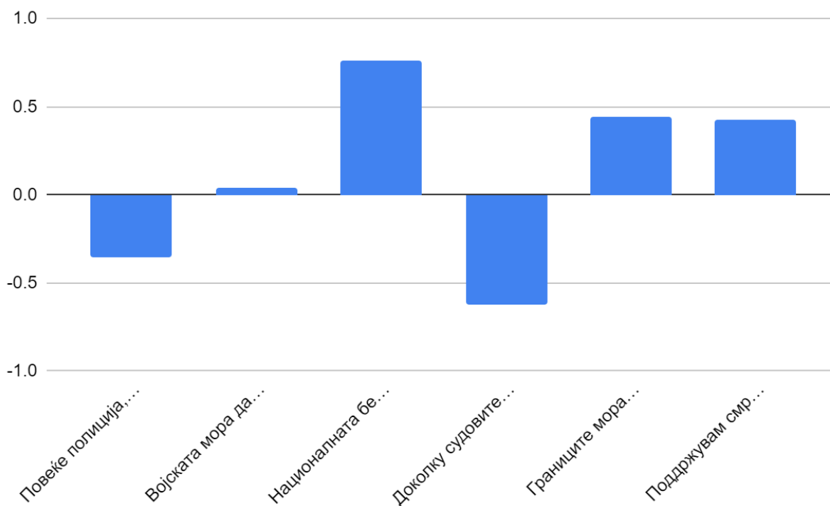
Графикон 9: Приказ на у вредности во безбедносно-правосудна функција
