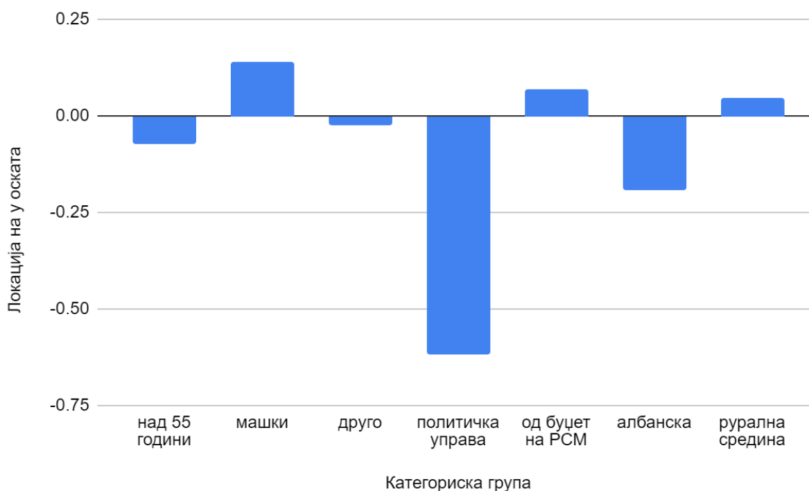
Графикон 17: Приказ на у вредности на категориски групи со нај-врховистички позиции
