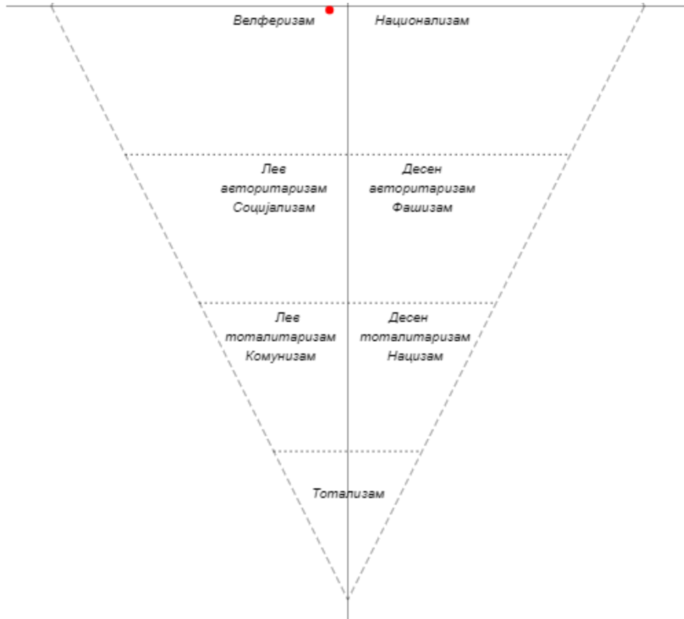
Слика 75: Графички приказ на долен триаголник на идеолошко каро за испитаници кои работаат во угостителство ( X = -0.0616 , Y = -0.0129 )
