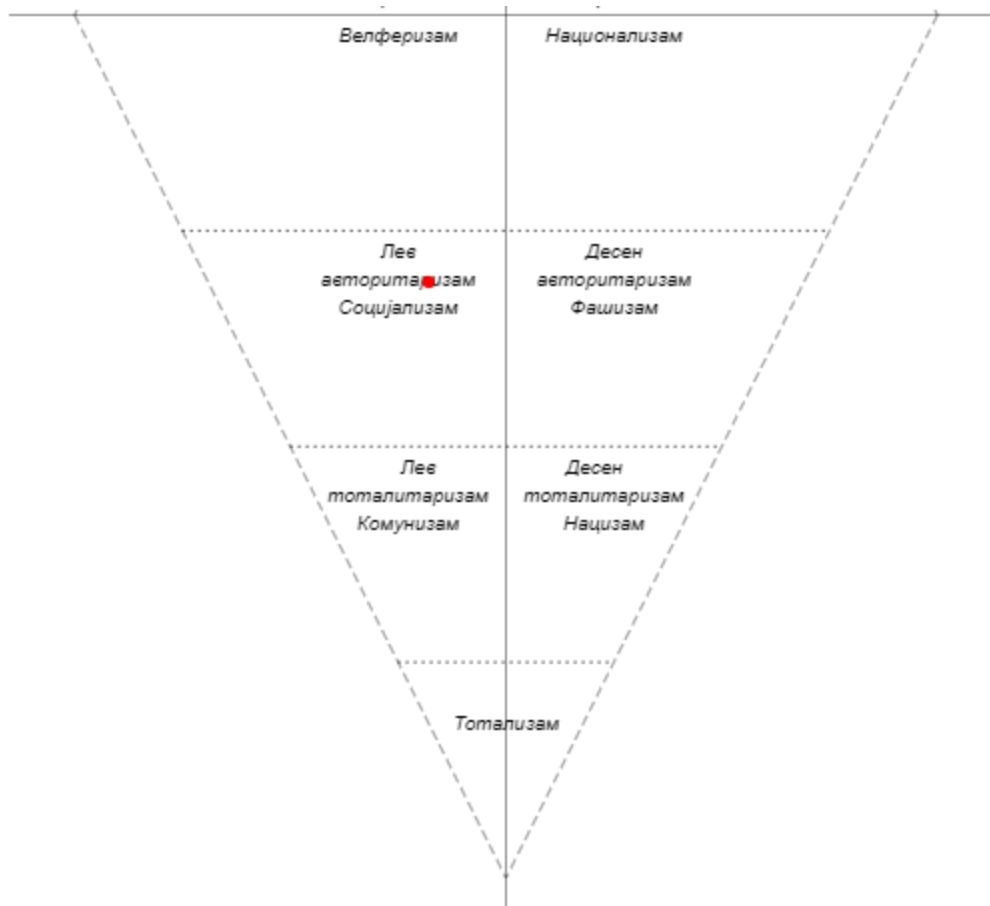
Слика 67: Графички приказ на долен триаголник на идеолошко каро за испитаници кои работаат во политичка управа ( X = -0.1785 , Y = -0.619 )
