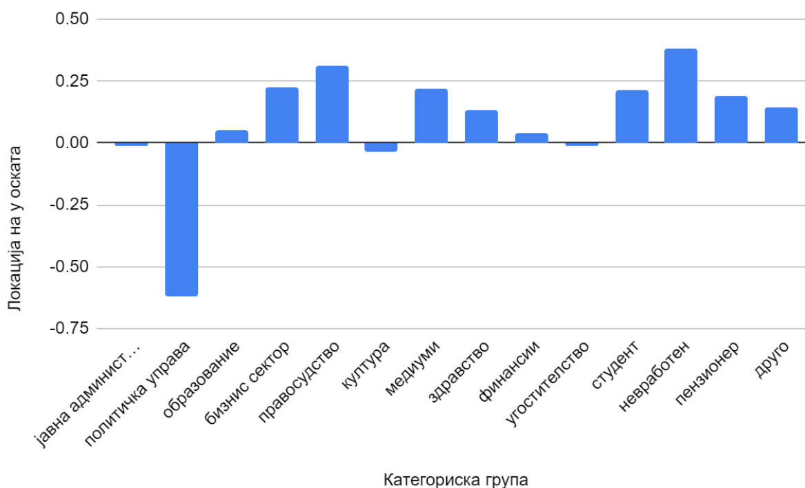
Графикон 4: Приказ на у вредности на испитаниците, според категорија работа
