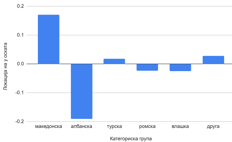
Графикон 6: Приказ на у вредности на испитаниците, според категорија етничка заедница
