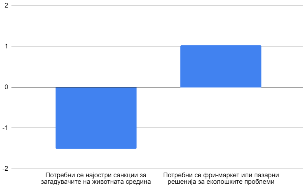
Графикон 14: Приказ на у вредности во еколошка функција
