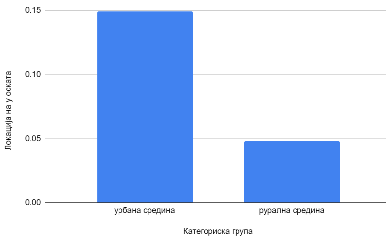
Графикон 7: Приказ на у вредности, според категорија место на живеење
